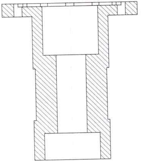
SECCIÓN A-A
