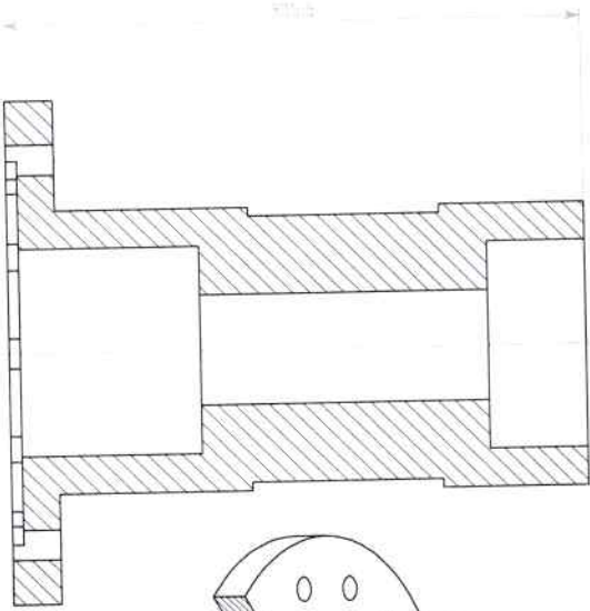
SECCIÓN B-B
