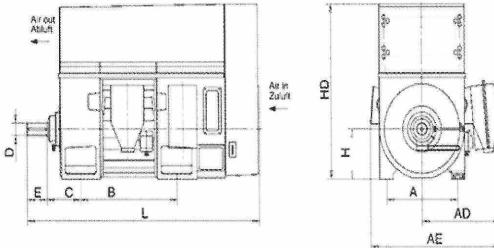
Maßbild 3
