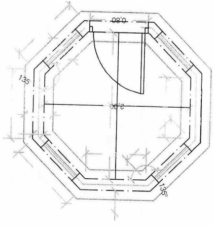
CIMIENTOS
