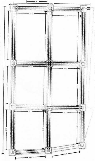
PLANO CIMIENTOS
