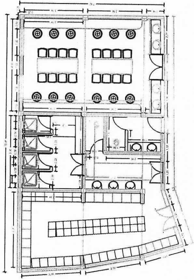
PLANO PLANTA ALTA
