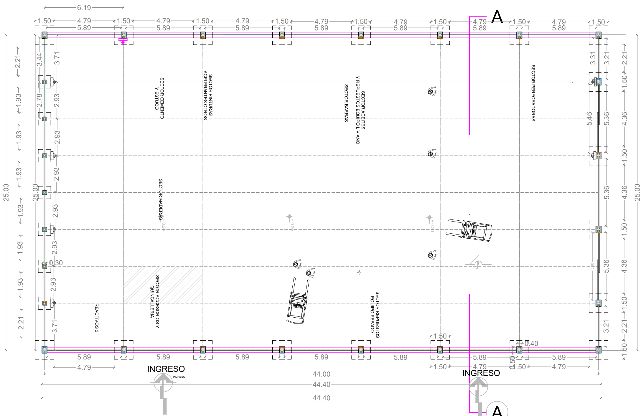
PLANO DE CIMIENTOS
