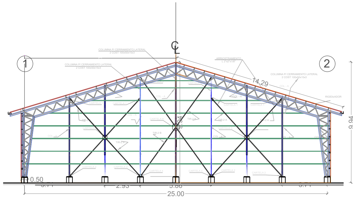
ESTRUCTURA METALICA PORTANTE (Item TEM-001)
