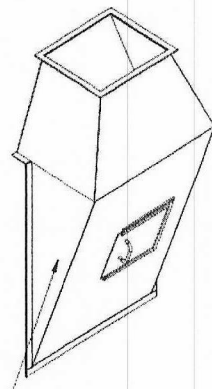
Vista B Escala 1:10 Todo el Material es ACERO INOXIDABLE Espesor de Plancha 1/4"
