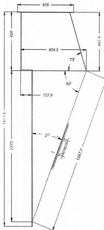
Vista B Escala 1:10 Todo el Material es ACERO INOXIDABLE Espesor de Plancha 1/4"
