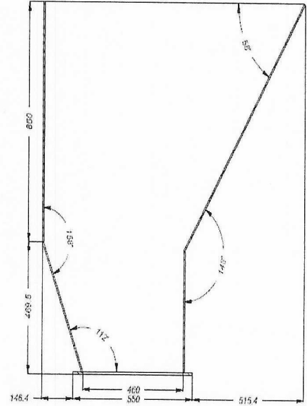
Sección C Escala 1:10
