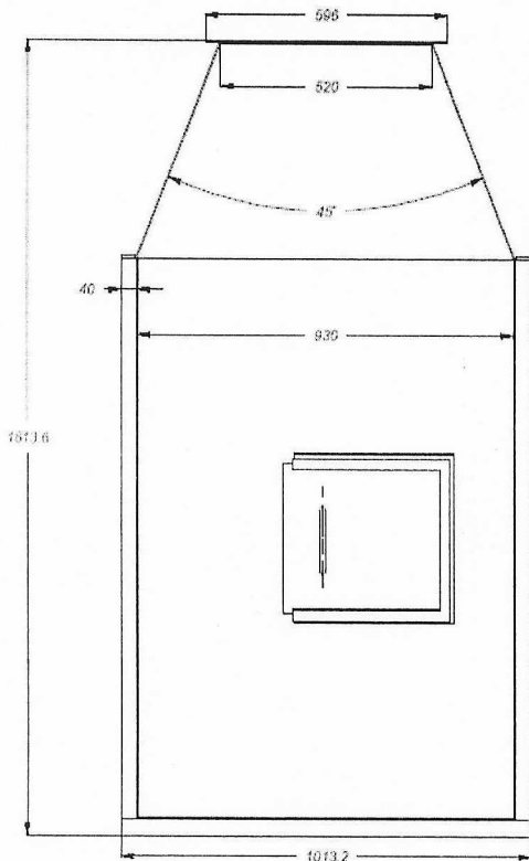
Vista A Escala 1:10
