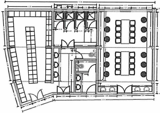
PLANO PLANTA ALTA
