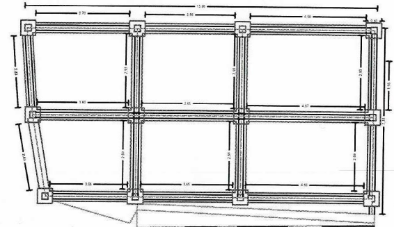
PLANO CIMIENTOS
