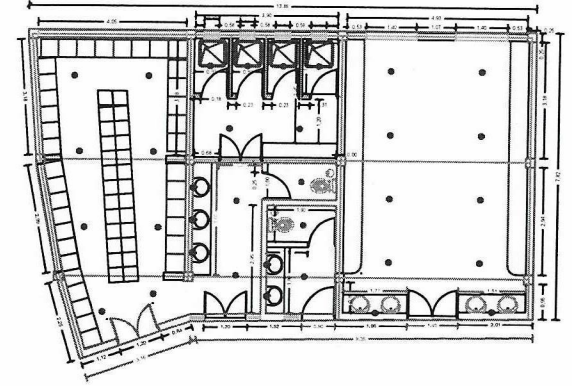
INSTALACION ELECTRICA
