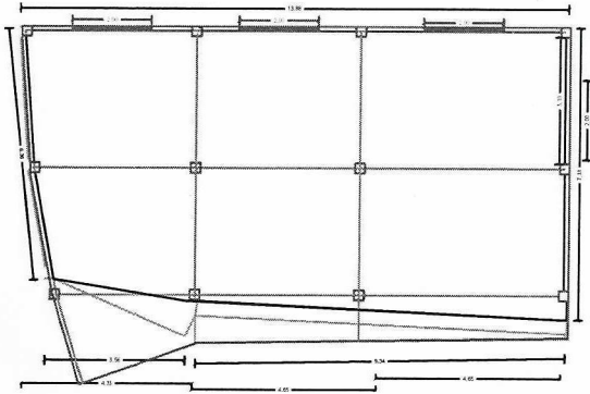
PLANO EN PLANTA BAJA
